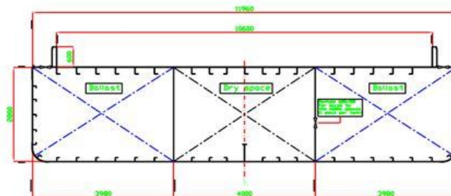
Transverse section - scale 1 : 50 -
